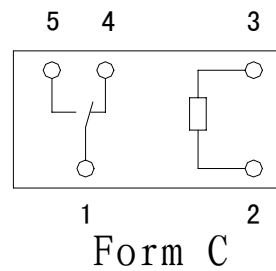
接线图
